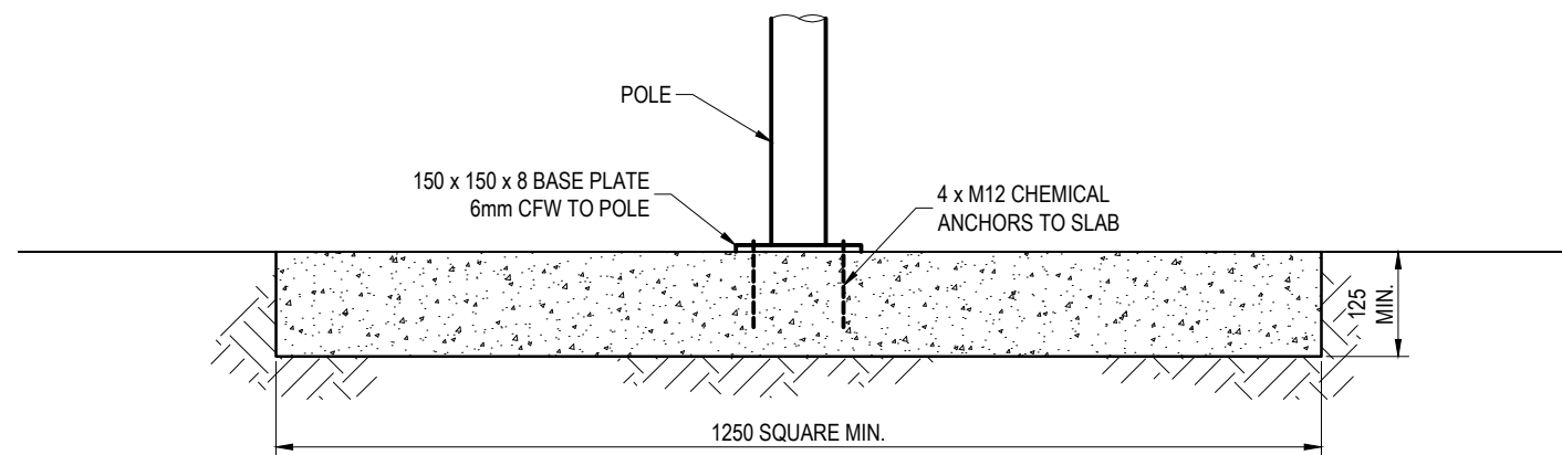
ELEVATION
