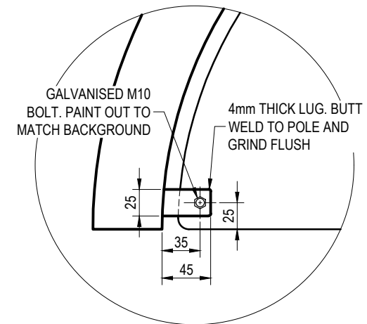
LUG DETAIL
