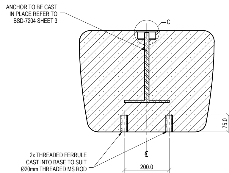
SECTION D-D
